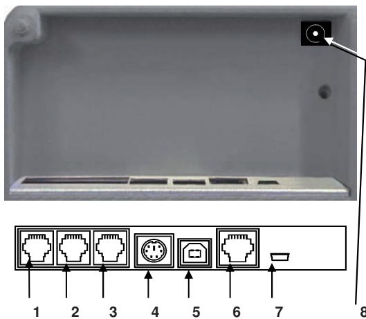
2. ábra - Csatlakozók a pénztárgép alján
